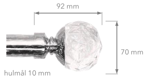
hulmål 10 mm
